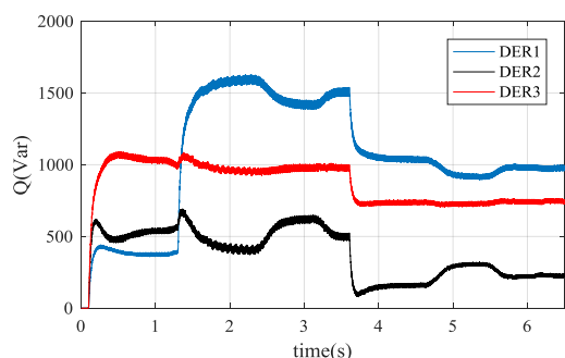
شکل ۱۹. منحنی توان راکتیو واحدهای DER (سناریو سوم)
