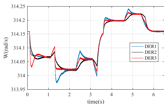
شکل ۱۷. منحنی فرکانس زاویه‌ای سیستم (سناریو سوم)
