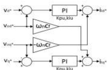
شکل ۲. حلقه کنترل ولتاژ
