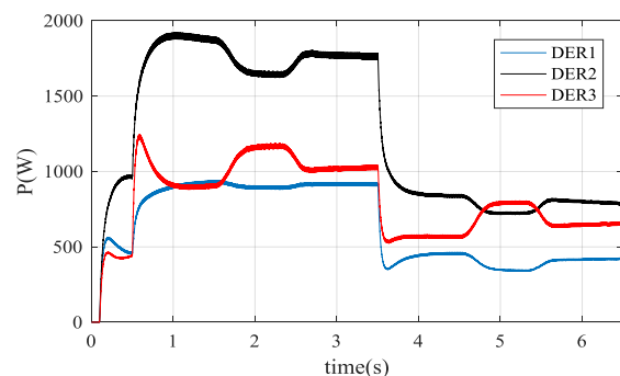
شکل ۱۳. منحنی توان اکتیو واحدهای DER (سناریو دوم)
