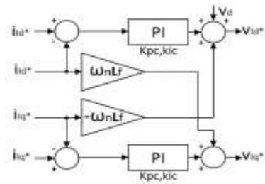
شکل ۳. حلقه کنترل جریان
