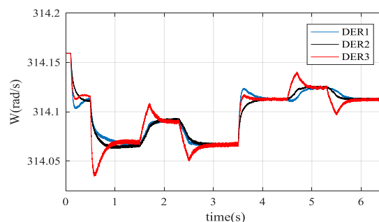
شکل ۱۲. منحنی فرکانس زاویه‌ای سیستم (سناریو دوم)
