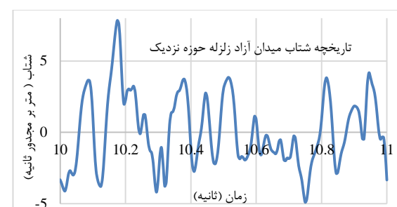
شکل ۲۶. مقایسه تاریخچه شتاب مقیاس شده به g میدان آزاد زمین سخت (تیپ I) برای انفجار مدفون و زلزله حوزه نزدیک (Landers) بزرگ‌نمایی شده برای زمان یک ثانیه
