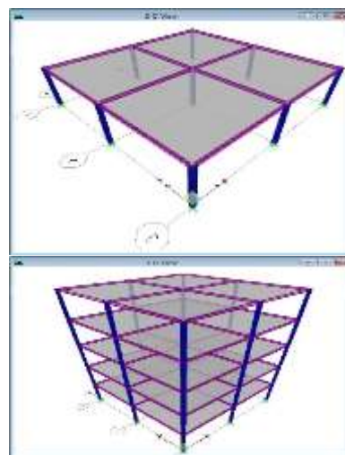
شکل ۳۰. تصویر مدل سازه یک و پنج طبقه در نرم‌افزار ETABS
