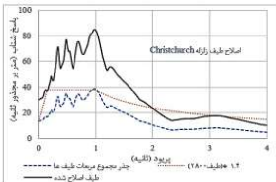
شکل ۷. اصلاح طیف زلزله ها با طیف آئین نامه ۲۸۰۰ زلزله
