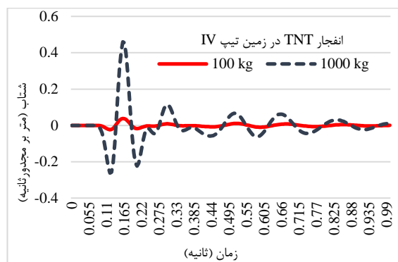
شکل ۲۱. نمودار مقایسه تاریخچه شتاب میدان آزاد زمین نرم در اثر
