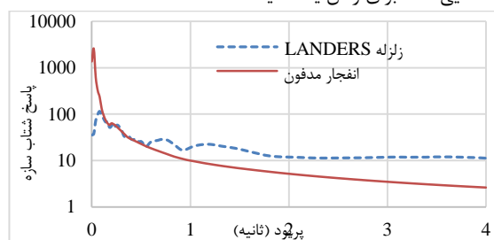
شکل ۲۷. مقایسه طیف‌های پاسخ شتاب سازه اصلاح‌شده با طیف آئین- نامه ۲۸۰۰ تحت اثر بارگذاری انفجار مدفون و زلزله حوزه نزدیک زمین سخت (تیپ I)
