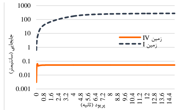
شکل ۱۳. نمودار مقایسه طیف پاسخ تغییر مکان سازه در اثر انفجار ۱۰۰ کیلوگرم ماده منفجره TNT در عمق ۱۵ متری زمین سخت و نرم
