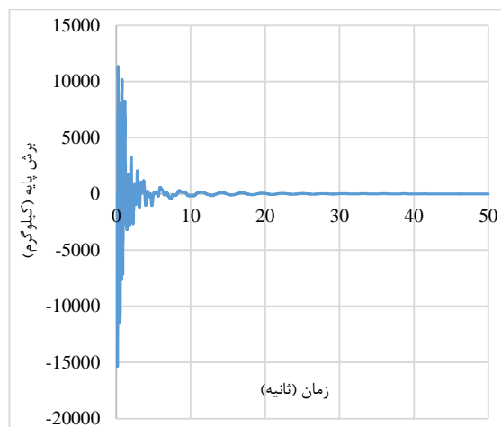
شکل ۳۷. نمودار تاریخچه برش پایه سازه پنج‌طبقه تحت انفجار مدفون در زمین نرم
