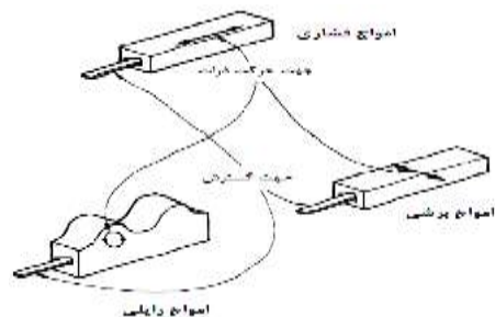
شکل ۱. حرکت ذرات و امواج فشاری، برشی و ریلی [۱۴]
