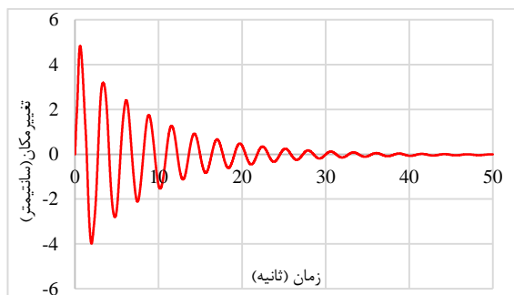
شکل ۳۵. نمودار تاریخچه تغییر مکان مرکز جرم دیافراگم طبقه آخر سازه پنج‌طبقه در اثر انفجار مدفون در زمین سخت
