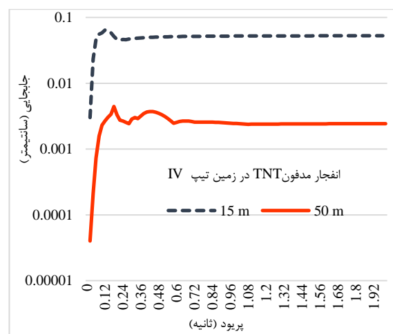
شکل ۱۸. نمودار مقایسه طیف پاسخ تغییر مکان سازه در اثر انفجار ۱۰۰ کیلوگرم ماده منفجره TNT در عمق ۱۵ و ۵۰ متری خاک نرم
