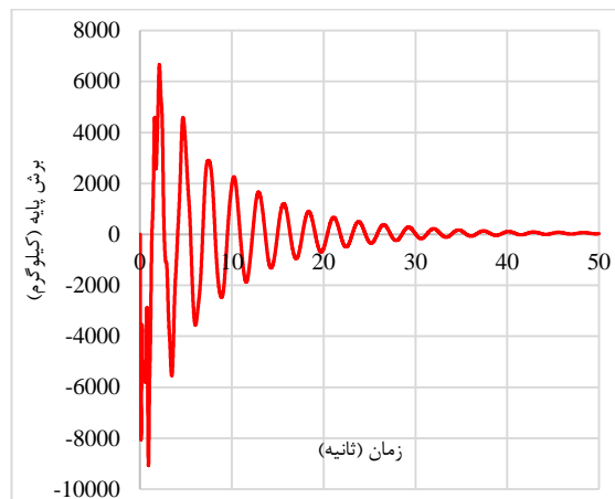
شکل ۳۶. نمودار تاریخچه برش پایه سازه پنج‌طبقه تحت انفجار مدفون در زمین سخت
