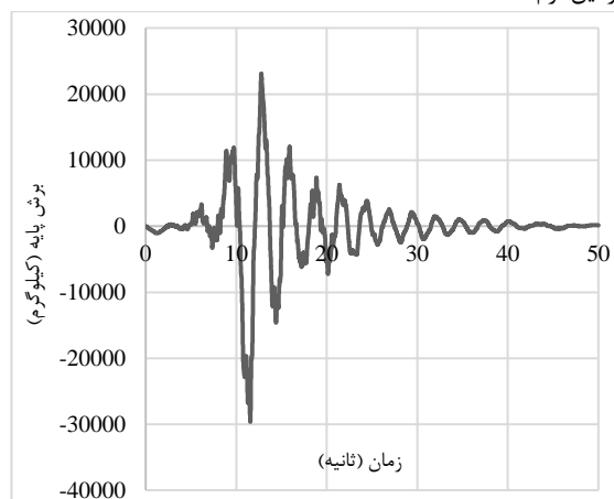
شکل ۳۸. نمودار تاریخچه برش پایه سازه پنج‌طبقه تحت زلزله زمین سخت LANDERS
