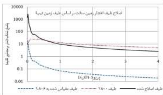
شکل ۶. اصلاح طیف های انفجار با طیف آئین نامه ۲۸۰۰
