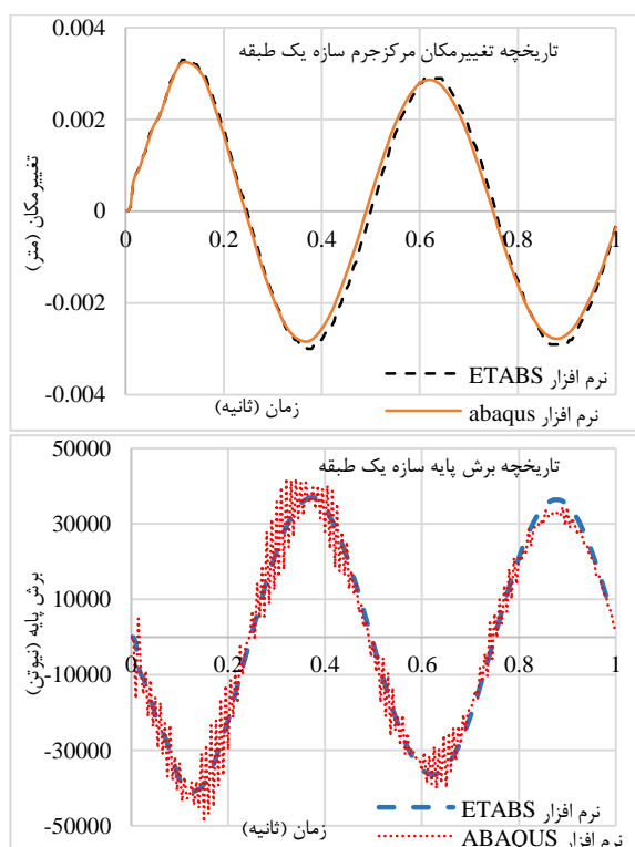
شکل ۱۰. تاریخچه تغییر مکان مرکز جرم دیافراگم و برش پایه سازه یک طبقه در اثر تحلیل تاریخچه زمانی رکورد انفجار توسط دو نرم‌افزار Etabs و ABAQUS [۱۶ و ۲۳]
