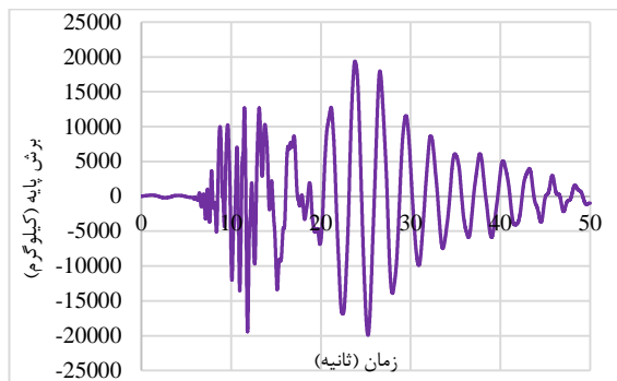
شکل ۳۴. نمودار تاریخچه برش پایه سازه پنج‌طبقه تحت زلزله زمین نرم CHRISTCHURCH
