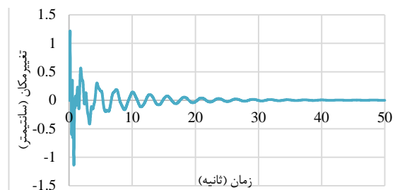
شکل ۳۶. نمودار تاریخچه تغییر مکان مرکز جرم دیافراگم طبقه آخر سازه پنج طبقه در اثر انفجار مدفون در زمین نرم
