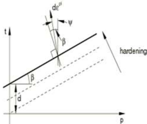
شکل ۳. سطح تسلیم و سخت‌شوندگی در مدل دراگر-پراگر [۱۶]
