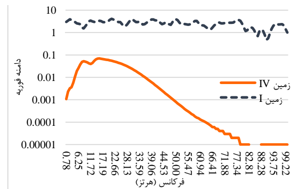
شکل ۱۴. نمودار مقایسه طیف فوری انفجار ۱۰۰ کیلوگرم ماده منفجره TNT در عمق ۱۵ متری زمین سخت و نرم
