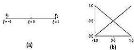
شکل ۲. المان خطی در نظر گرفته شده (a) هندسه المان (b) توابع شکل
