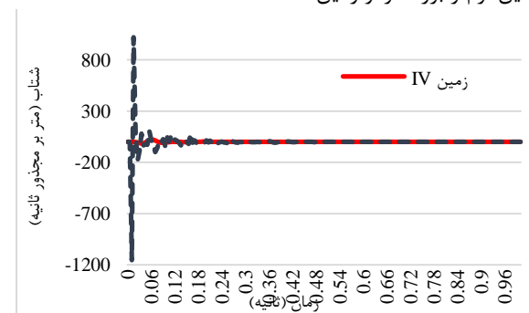
شکل ۱۵. نمودار مقایسه تاریخچه شتاب میدان آزاد انفجار ۱۰۰۰ کیلوگرم ماده منفجره TNT در عمق ۱۵ متری زمین سخت و نرم
