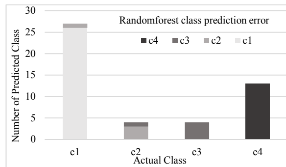
شکل ۱۵. نمودار خطای پیش‌بینی طبقه‌بندی‌کننده تقویتی انطباقی برای سیستم ۳۹ شین
