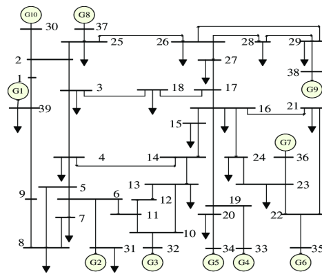
شکل ۱۲. دیاگرام تک خطی شبکه ۳۹ شینه استاندارد
