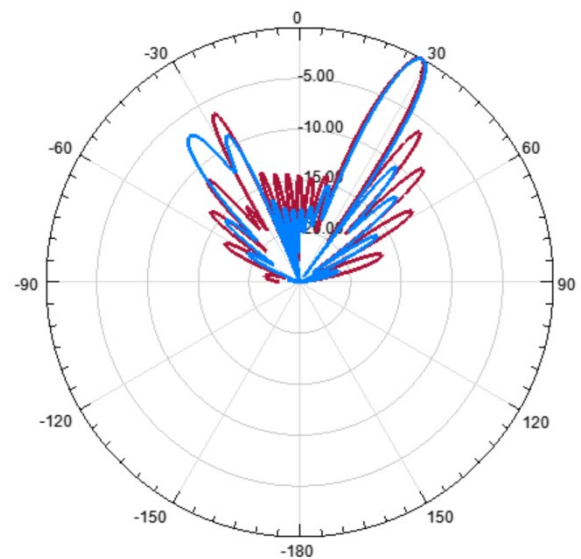
شکل ۲. نمودار تشعشعی حاصل از امپدانس سطحی مربعی (آبی) و امپدانس سطحی سینوسی (قرمز)
