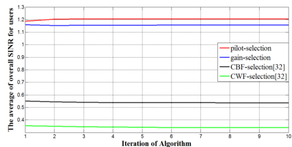
شکل ۷. میانگین مجموع SINR هر کاربر در آنتن‌های گروهی خود برای روش‌های انتخاب آنتن مختلف
