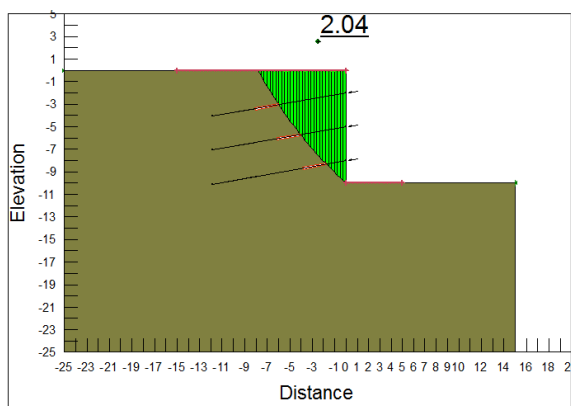
شکل ۱۵. مدل چهارم (تماماً انکر (۲)) در نرم‌افزار GeoStudio
