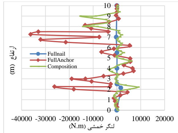
شکل ۹. لنگر خمشی در شاکریت
