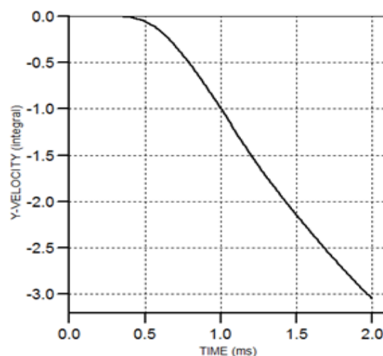
شکل ۹. جابجایی نقطه ۳ با قرارگیری مواد ناریه در فاصله ۱ متر
