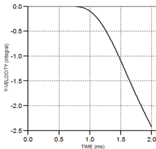
شکل ۱۱. جابجایی نقطه ۳ با قرارگیری مواد ناریه در فاصله ۲ متر
