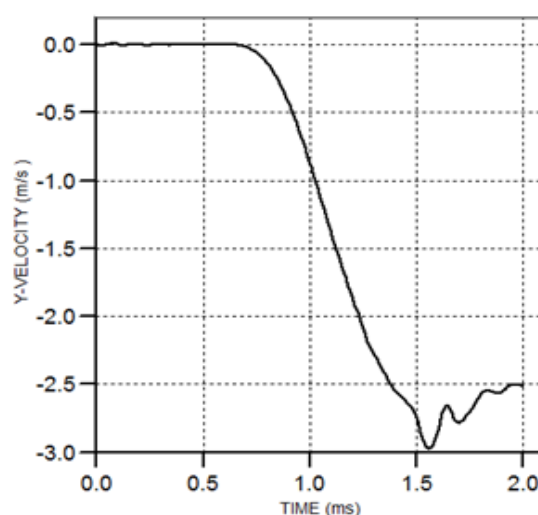
شکل ۱۰. سرعت حرکت نقطه ۳ در واحد زمان با قرارگیری مواد ناریه در فاصله ۲ متر
