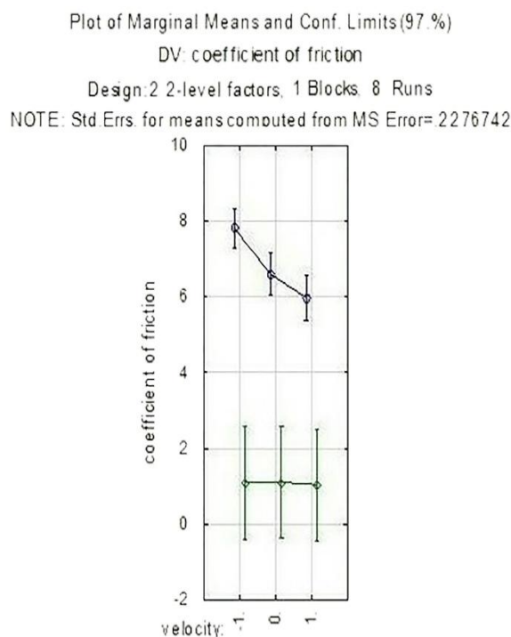
شکل ۸. خطوط دو بعدی ضرایب اصطکاک الیاف خام و آغشته شده به STF
