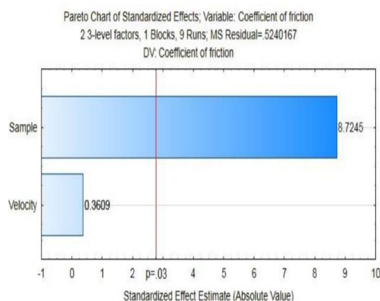
شکل ۹. نمودار پارتو نشان‌دهنده تأثیر متغیرها بر نتایج آزمون بیرون‌کشی الیاف.
