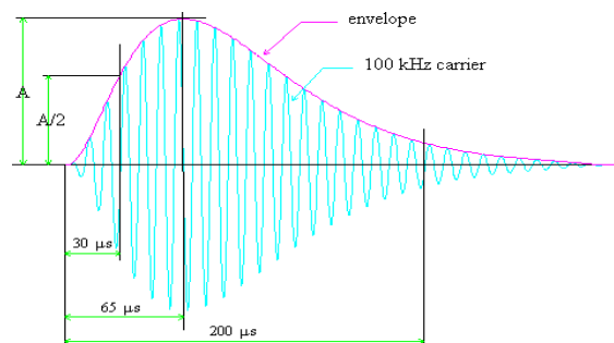
شکل ۳. ساختار پالس لورن [۱]
