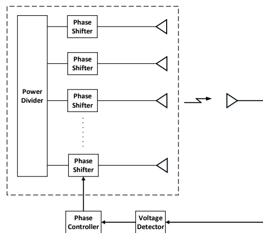
شکل ۴. ساختار روش ارائه شده برای آنتن آرایه فازی در مد ارسال
