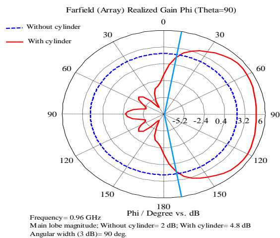
شکل ۲۱. پترن Azimuth
