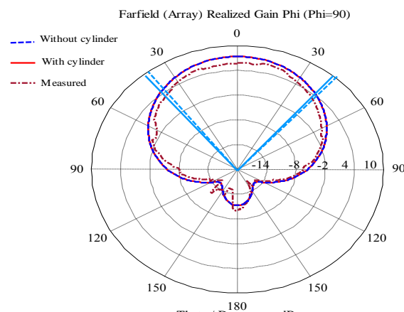
شکل ۱۴. پترن Co-Polar
