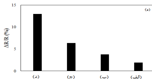
شکل ۱۱. نمودار پاسخ حسگر لایه نشانی شده با گرافن اکساید احیا شده توسط (الف) گلوکز، (ب) آسکوربیک اسید، (ج) هیدرازین هیدرات، (د) PPD در غلظت ۲/۵ mg/L برای بخارات مختلف (ه) مقایسه نتایج پاسخ حسگرهای الف تا د برای DMMP
