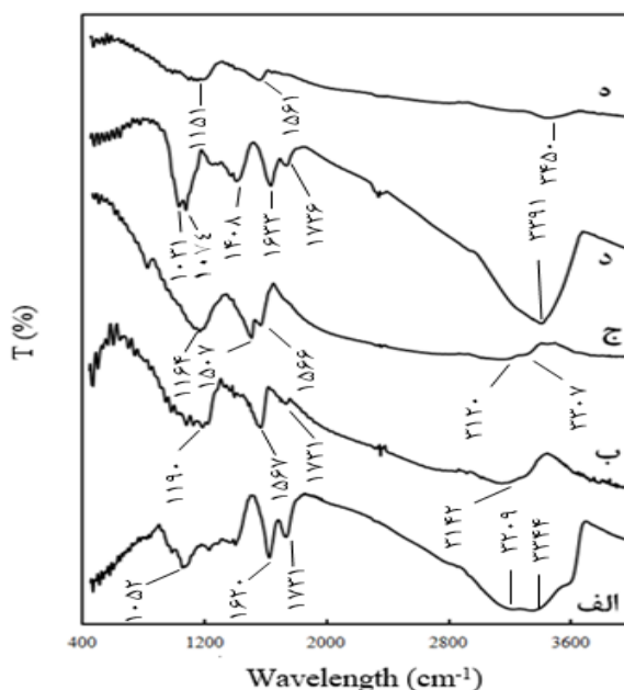
شکل ۴. طیف‌های FT-IR گرافن اکساید (الف)، گرافن اکساید احیا شده با اسیدآسکوربیک (ب)، پارافنیل دی‌آمین (ج)، با گلوکز (د) و با هیدرازین هیدرات (ه)
