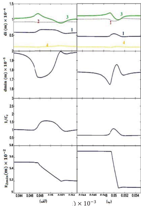
شکل ۱۶. اثرات مکان عدسی کر L_{2k} بر روی پارامترهای باریکه. پارامترهای شکل (۱۴) به استثناء L_{23}=113.2mm (ناحیه II).
