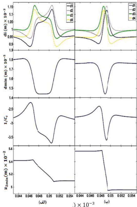
شکل ۵. اثرات مکان عدسی کر L_{2k} بر روی پارامترهای باریکه. تشدیدگر متقارن ( L_{12}=L_{34} ) برای ناحیه I با L_{23}=105.2\text{mm} و P=2 \times 10^3 .
