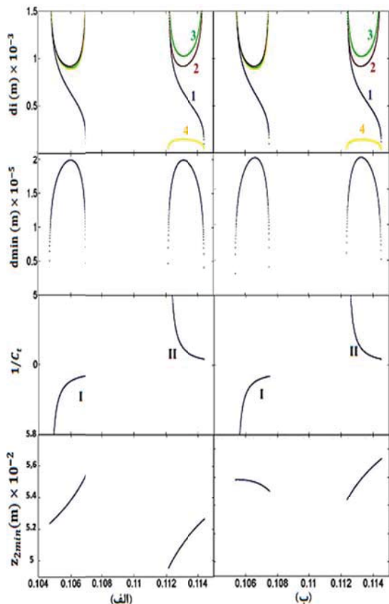
شکل ۴. پارامترهای باریکه برای تشدیدگر نامتقارن ( L_{12}=3L_{34} ) با خنثی کردن آستیگماتیسم و بدون در نظر گرفتن عدسی کر ( p=0 ). مرکز صفحه بروستر در ( l_{23}/2 ) می باشد. پارامترهای جدول ۲ به کار گرفته شده است. (الف) محور عمودی (ب) محور مماسی.
