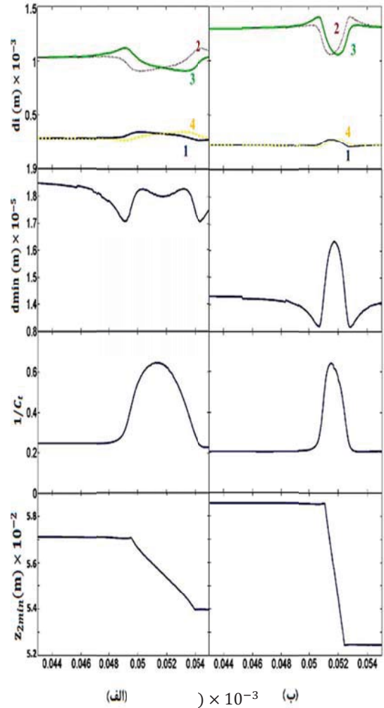
شکل ۱۳. اثرات مکان عدسی کر L_{2k} بر روی پارامترهای باریکه. پارامترهای شکل (۵) به استثناء L_{23}=111\text{mm} (ناحیه II).
