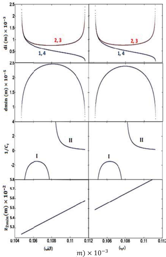
شکل ۳. پارامترهای باریکه برای تشدیدگر متقارن ( L_{12}=L_{34} ) با خنثی کردن آستیگماتیسم و بدون در نظر گرفتن عدسی کر ( p=0 ) در مرکز صفحه بروستر در ( l_{23}/2 ) می‌باشد. پارامترهای جدول (۲) به کارگرفته شده است. (الف) محور عمودی (ب) محور مماسی.
