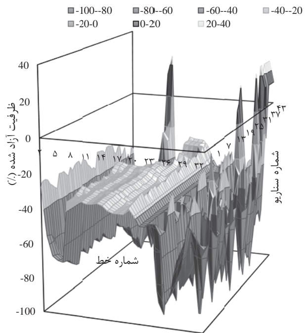
شکل ۱۲. ظرفیت آزاد شده خطوط (ترکیب بهینه منابع انرژی)
