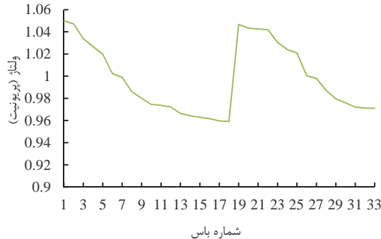
شکل ۸. پروفیل ولتاژ مورد انتظار شبکه (حالت پایه)
