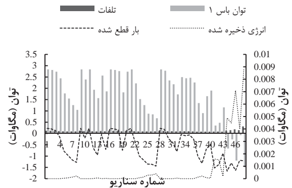
شکل ۱۵. تلفات توان، توان باس ۱، بار قطع شده و توان مازاد در هر سناریو
