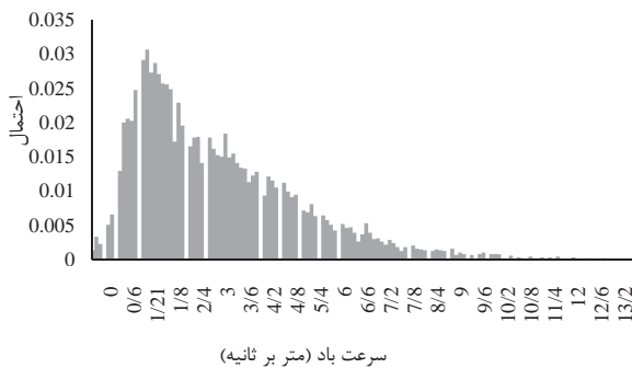
شکل ۱. تابع چگالی احتمال سرعت باد [۲۲]
