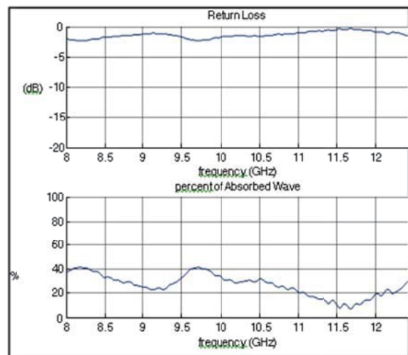
شکل ۶. اتلاف امواج رادار توسط کامپوزیت پلی‌یورتان، پلی‌آنیلین با ضخامت ۴ میلی‌متر برای کامپوزیت در شرایط غلظتی ۴۰ درصد (وزنی/وزنی)، نمودار بالا، افت انعکاس توان موج برگشتی (برحسب dB) و نمودار پایین، جذب به صورت درصد
