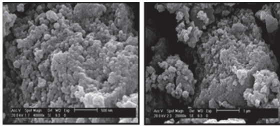
شکل ۴. تصویر میکروسکوپی الکترونی نانوذرات اکسید تیتان با ساختار تقریباً گروی با اندازه متوسط ۸۰-۴۰ نانومتر
