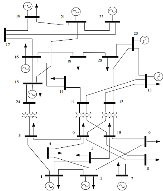
شکل ۲. شبکه آزمایش ۲۴ باس IEEE
