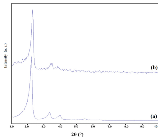
شکل ۳. تصویر XRD سیلیکای نانومتخلخل (a) MCM-41 و (b) NH 2 -MCM-41
