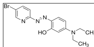
شکل ۱. ساختار Br-PADAP [۱۰]
