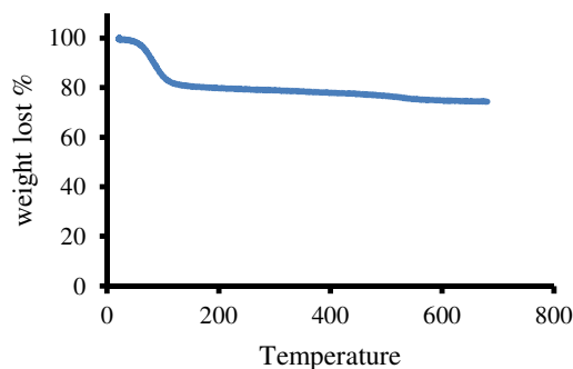
شکل ۵. تصویر TGA سیلیکای نانومتخلخل NH 2 -MCM-41
