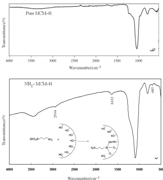
شکل ۴. تصویر اسپکتروسکوپی FT-IR سیلیکای نانومتخلخل MCM-41 (الف) و NH 2 -MCM-41 (ب)
