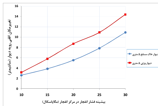
شکل ۷. مقایسه بیشینه تغییر مکان افقی دو نوع دیوار ۵ متری در برابر بیشینه فشار انفجار
