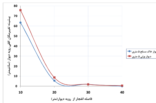
شکل ۹. مقایسه بیشینه تغییر مکان افقی دو نوع دیوار ۵ متری
