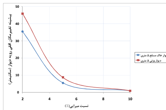
شکل ۸. مقایسه بیشینه تغییر مکان افقی دو نوع دیوار ۵ متری در برابر تغییرات نسبت میرایی
