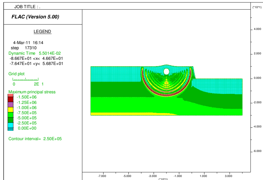
شکل ۵. لحظه رسیدن موج تنش انفجار به دیوار - ثانیه ۰/۰۵۵
