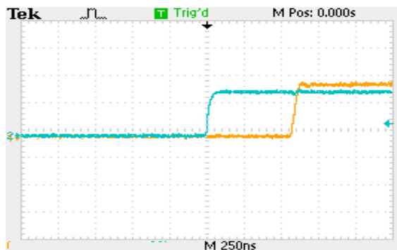
شکل ۱۵. تاخیر زمانی کل سامانه برابر ۵۷۵ نانوثانیه. سیگنال آبی پررنگ: سیگنال فرمان به فرستنده و سیگنال نارنجی - کم‌رنگ: سیگنال خروجی گیرنده بعد از دروازه زمانی (این میزان مستقل از اندازه کاراکترها است).
