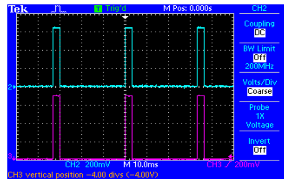
شکل ۱۴. سیگنال اعمالی به فرستنده (بنفش - پایین) و سیگنال دریافتی از خروجی گیرنده (سبز-بالا). که به خوبی تطابق ۱۰۰ درصدی سیگنال‌های ارسالی و دریافتی را نشان می‌دهد.
